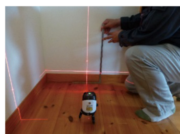
床の傾きの調査
